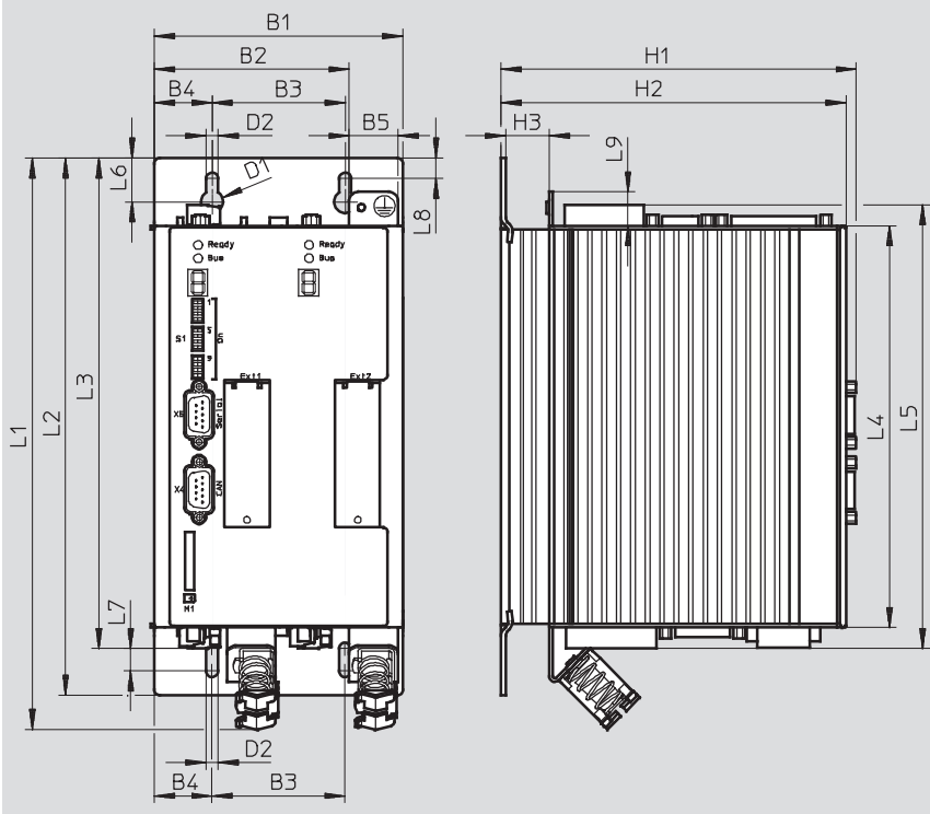
Dimensiones
