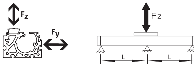
Fuerza Fz
