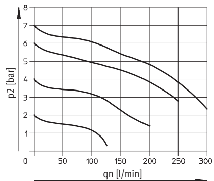
FRC-QS4-...-MICRO
