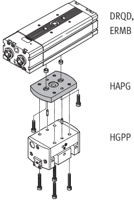
Montaje directo DRQD-...-FW en eje con brida ERMБ-... en eje de salida
