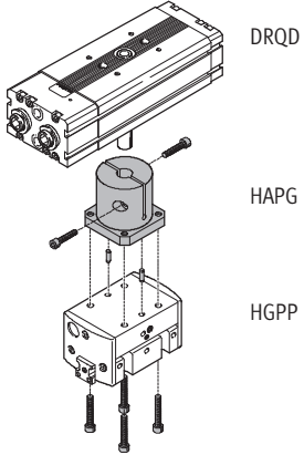
Montaje directo DRQD-...-ZW en eje con brida
