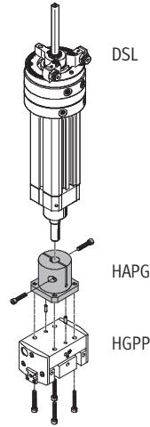
Montaje directo DSL-...-KF con eje con claveta
