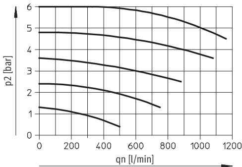
Caudal qn en función de la presión secundaria p2
