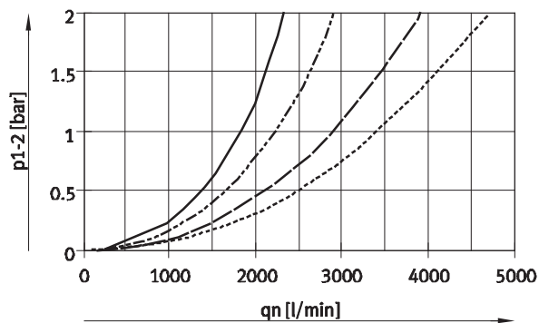
Caudal normal qn en función de la presión diferencial p1-2
