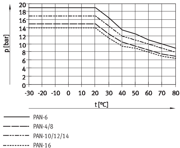
Presión de funcionamiento p en función de la temperatura t
