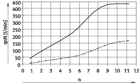
Caudal nominal normal qn con 6 bar → 0 bar en función de los giros n del husillo
