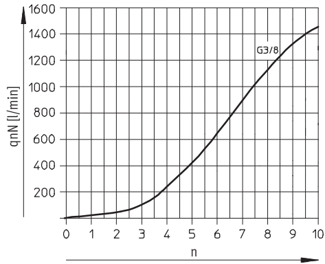
Caudal nominal normal q_{nN} con 6 bar \rightarrow 5 bar en función del giro n del husillo
