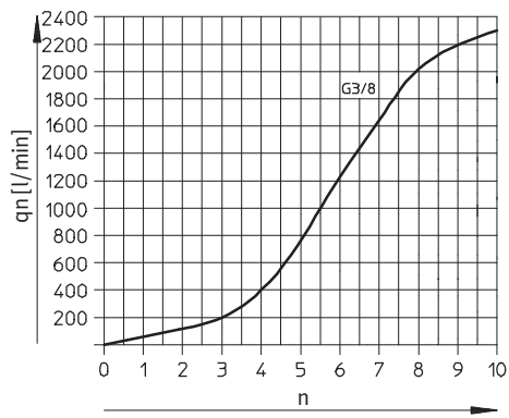
Caudal normal q_n con 6 bar \rightarrow 0 bar en función del giro n del husillo
