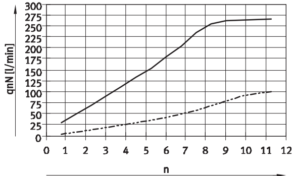
Caudal nominal normal qnN con 6 bar → 5 bar en función de los giros n del husillo
